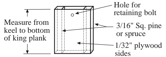
Fin Tongue
